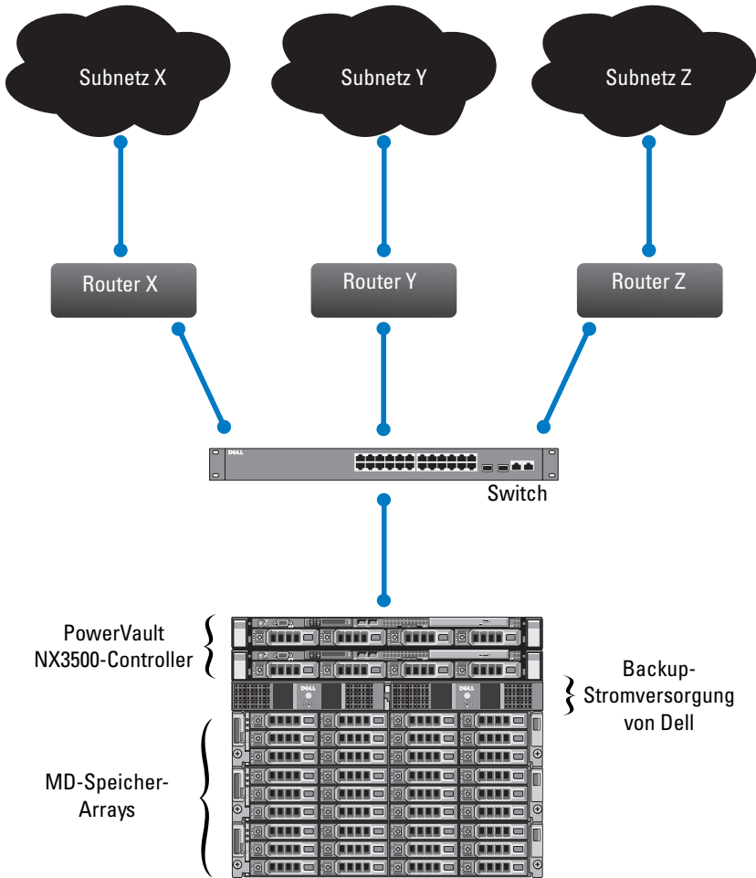
Abbildung 8-1. Netzwerkkonfiguration
